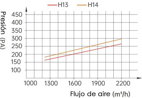
Diagrama de flujo de aire y resistencia 610*610*110
